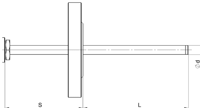
Рисунок А.12 – Термопреобразователи модификаций CTR, CTU с вынесением монтажной головки
