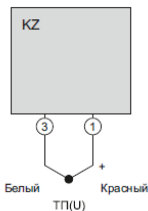
Рисунок 4 – Схема внешних электрических соединений термопреобразователей модификации СТU с оснащением монтажной головки KZ
