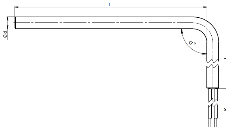
Конструктивное исполнение ВТ \alpha
