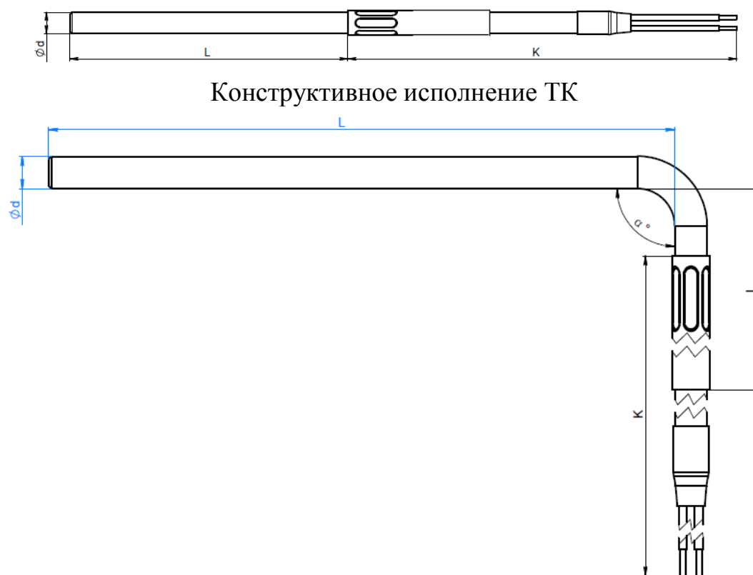
Конструктивное исполнение ТК \alpha
