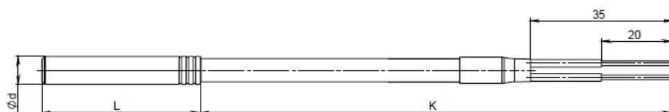
Конструктивное исполнение Е1
