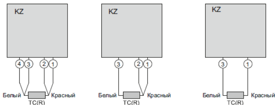
Рисунок 3 – Схема внешних электрических соединений термопреобразователей модификации СТР с оснащением монтажной головки KZ
