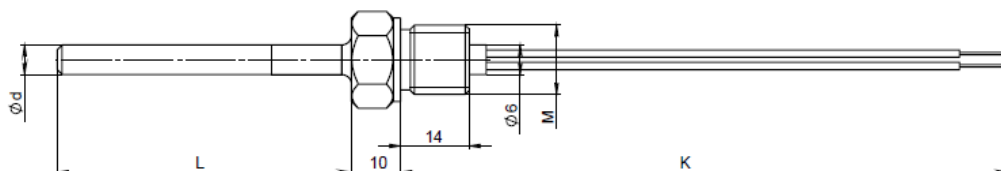
Конструктивное исполнение В
