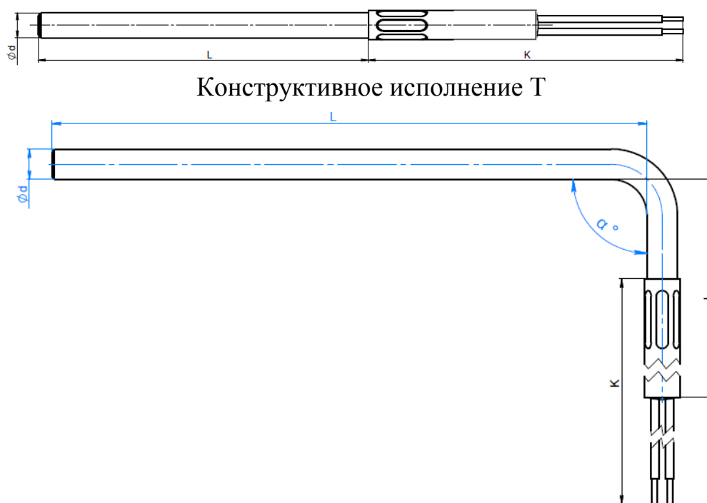
Конструктивное исполнение Та
