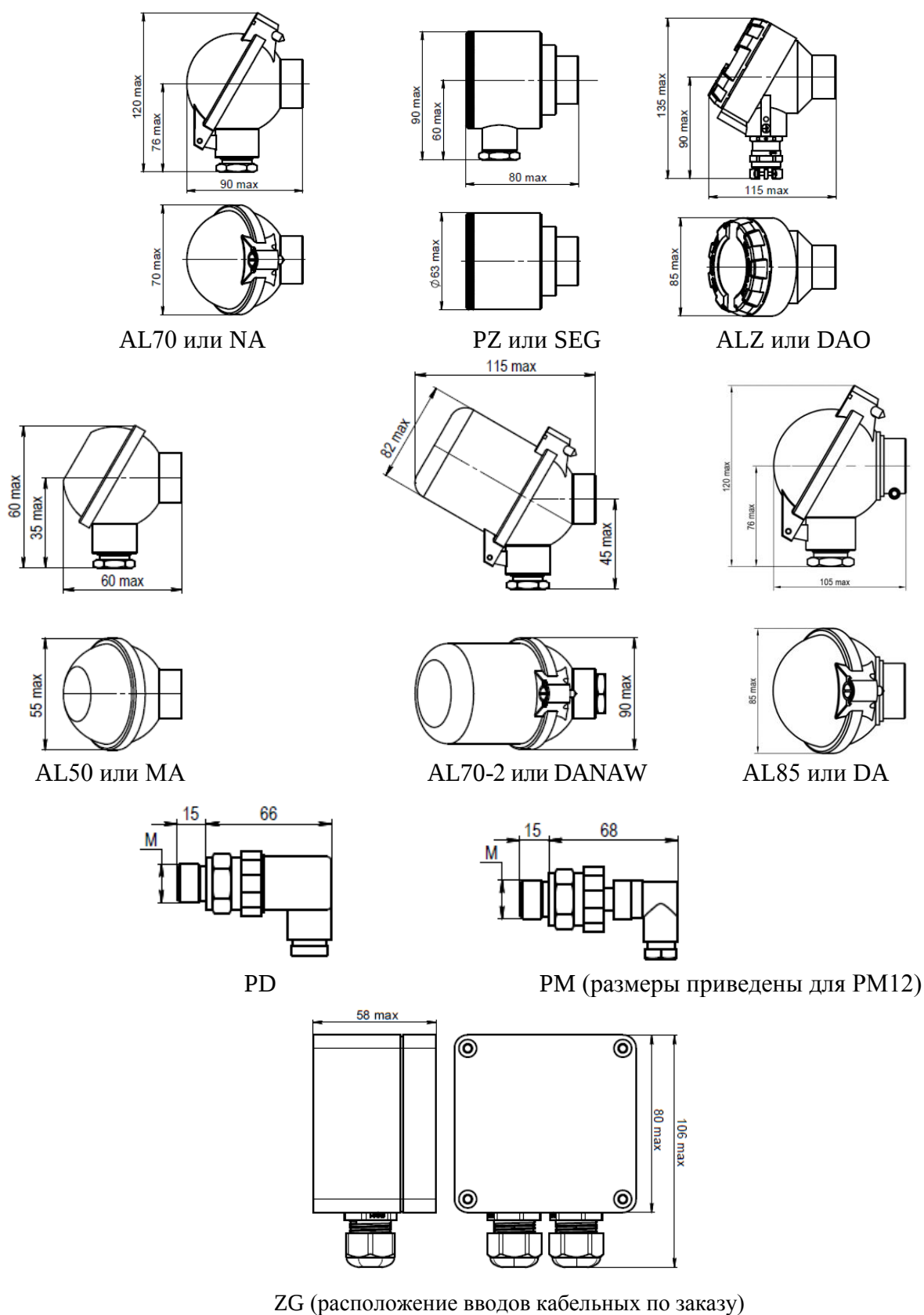
Рисунок А.9 – Монтажные головки из алюминия, нержавеющей стали и полимеров
